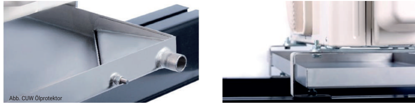
Abb. CUW Ölprotektor
